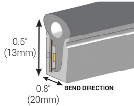
SCM-AL-NEON
